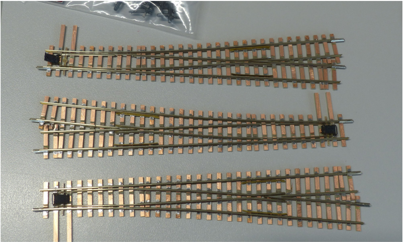
H0m Code 75 Hobby-Line 3 x EW 80 1:7 unlackiert mit Weichenverschlußdeckel
