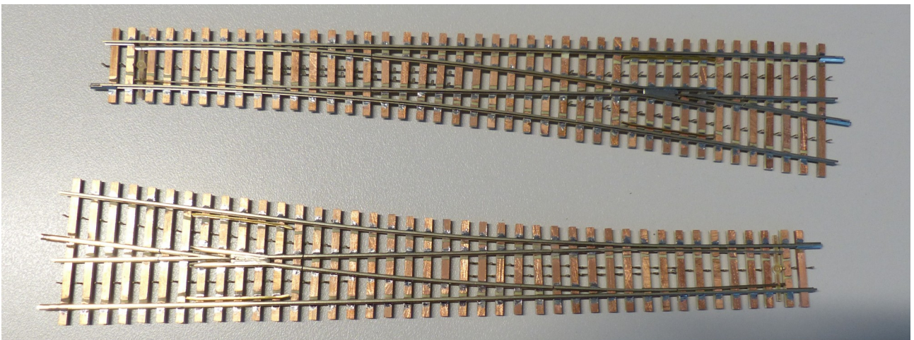
H0 3+2L Code 83 Hobby-Line zwei EW R 500/8°
